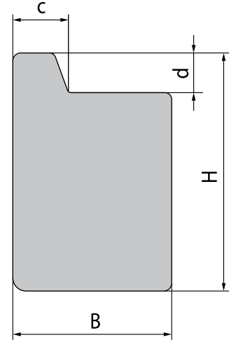
Querschnittsform Typ B Cross-section Type B
